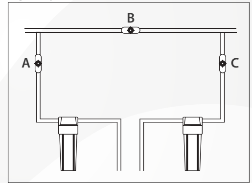
Fig. 2: By-Pass - Fontanería
